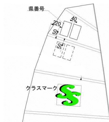
セーリングスピリッツ級ダクロンセー ル 県番号表示位置
