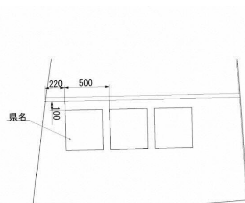
セーリングスピリッツ級マイラーセー ル 県番号・県名表示位置
