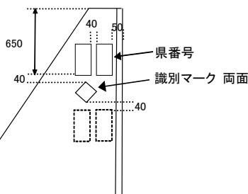
420級 県番号表示位置
