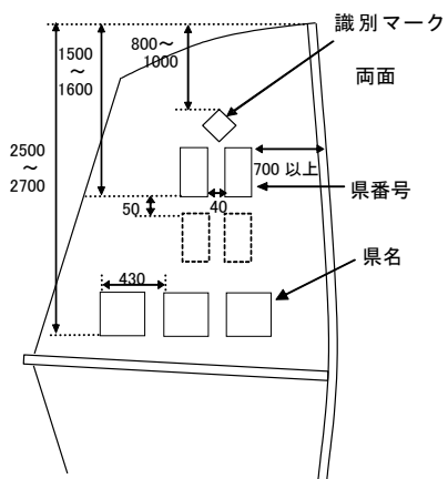
ILCA6級 県番号表示位置
